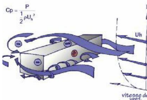
Le champ de pression induit par le vent sur les obstacles bâtis. Illustration : Livret PREBAT 3 ADEME - Jacques Gandemer
