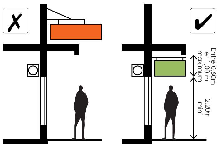
Coupes exemples sur devantures intégrées ou non à la volumétrie de la façade
