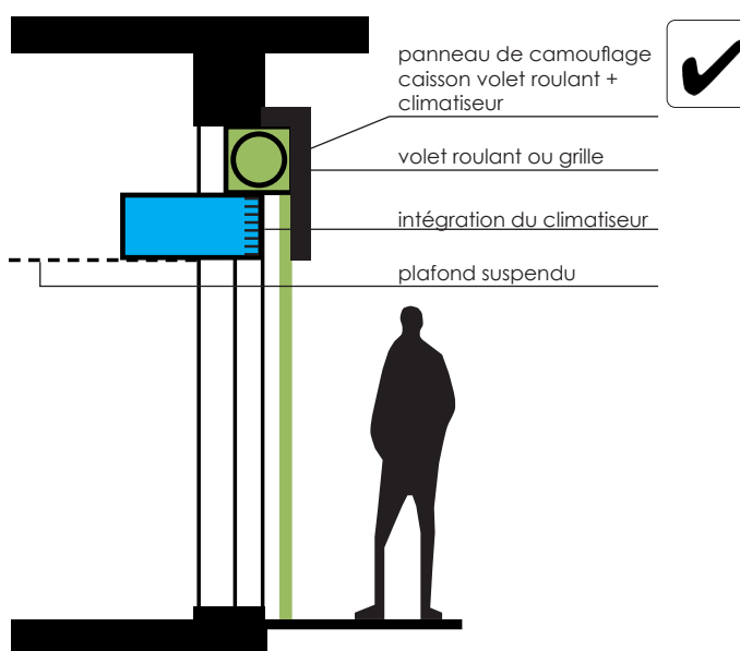
Exemples d'intégration du compresseur
