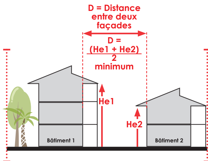
Schéma de principe du rapport hauteur/largeur entre bâtis D= distance entre les façades des corps de bâtis He1= Hauteur à l'égoût du bâtiment 1 He2= Hauteur à l'égoût du bâtiment 2
