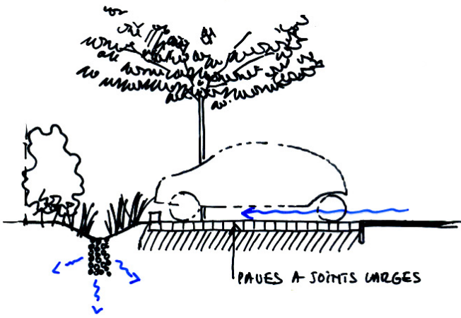
La noue en fond de parking facilite l'infiltration et participe au paysage du cœur d'îlot
