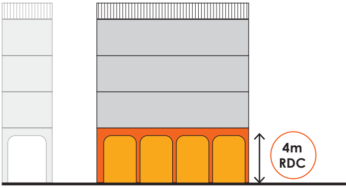
Élévation de façade type sur Avenue de la République : principe de la galerie en RDC sur une hauteur de 4m minimum
