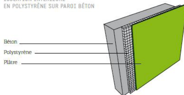
ISOLATION INTÉRIEURE EN POLYSTYRÈNE SUR PARI BIÉTON
